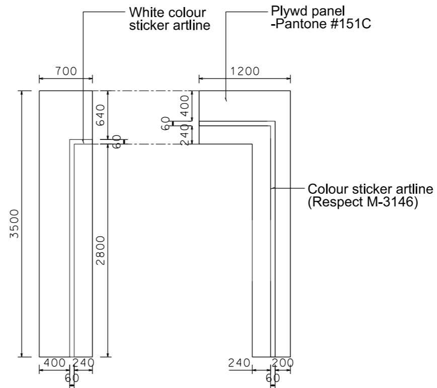
FASCIA ELEVATION
